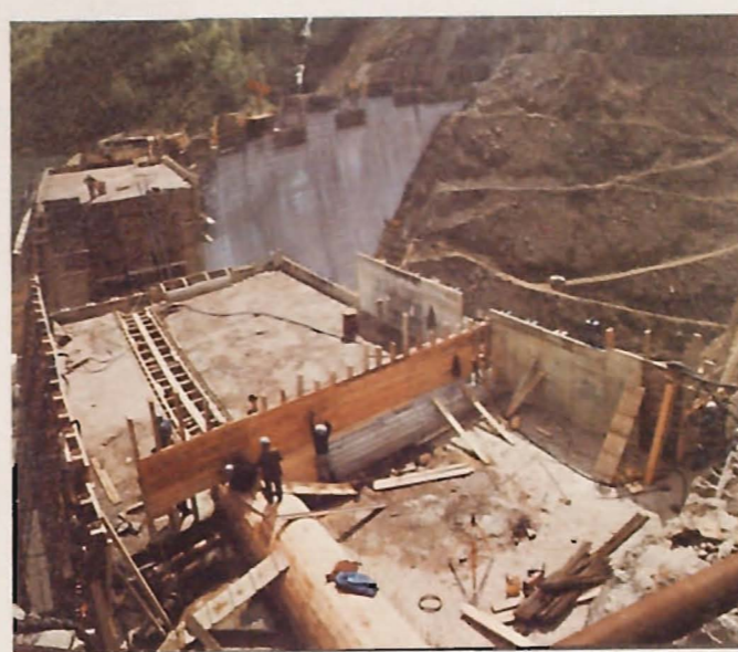
presa de Baserca. En construcción (30.5.1983)
